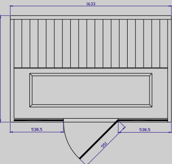
TYLÖSAND T-825 Mått: D 1078 x W 1633 Effekt: 1980 W
