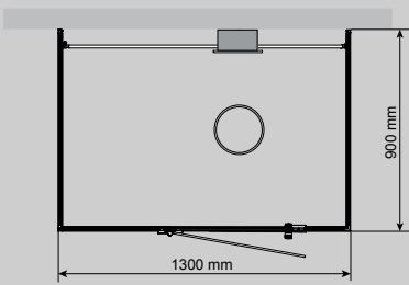
VISTA DCO 130 HÖGER Mått: D 900 x B 1300 mm
