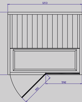
TYLÖSAND T-820 Mått: D 1 013 x B 1 213 mm Effekt: 1470 W
