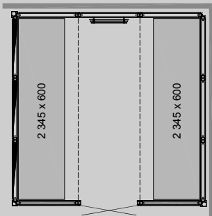
PANACEA 2525 2B Mått: 2 525 x 2 525 x 2 090 mm
