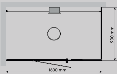
VISTA 160 HÖGER Mått: D 900 x B 1 600 mm
