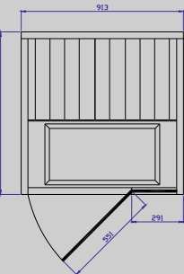
TYLÖSAND T-810 Mått: D 913 x B 913 mm Effekt: 1350 W
