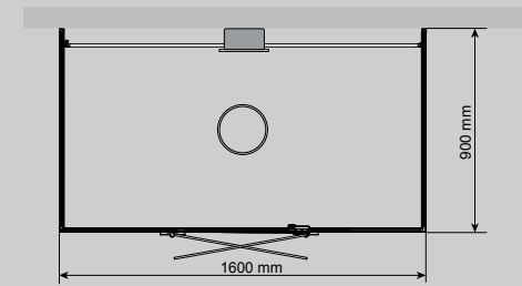
VISTA DCO 160 (VÄNSTER & HÖGER) Mått: D 900 x B 1 600 mm
