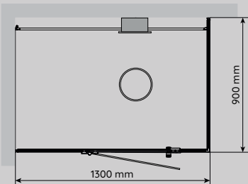
VISTA 130 HÖGER Mått: D 900 x B 1 300 mm
